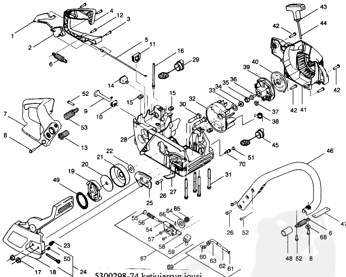
5300298-74 ketjujarrun jousi
