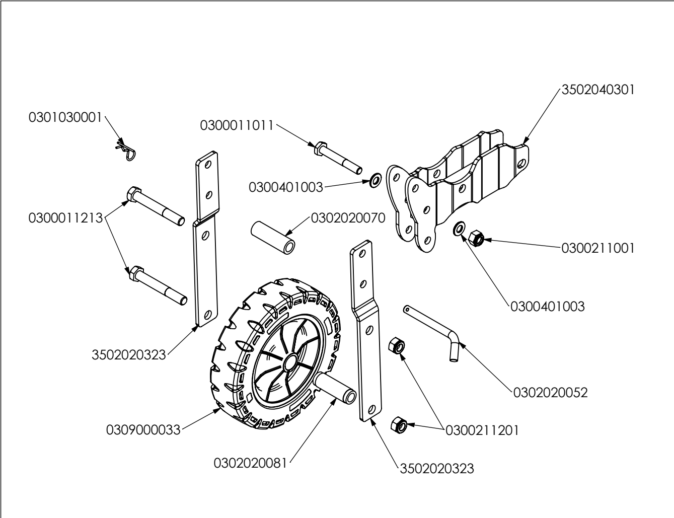
35_Roue transport QJV3 Défaut
